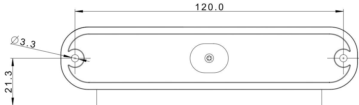
Rear view Scale: 1:1
